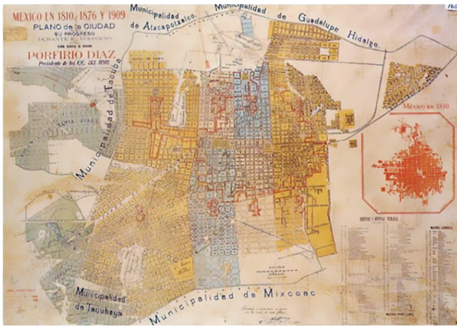
Figura 13. Sistema de Barrios de la Ciudad del Orden y Progreso, Ciudad de México 1810 (perímetros A y B) y Ciudad de Méxioco-1876-1909 (posible perímetro D del Centro Histórico o Ciudad del Interior).
